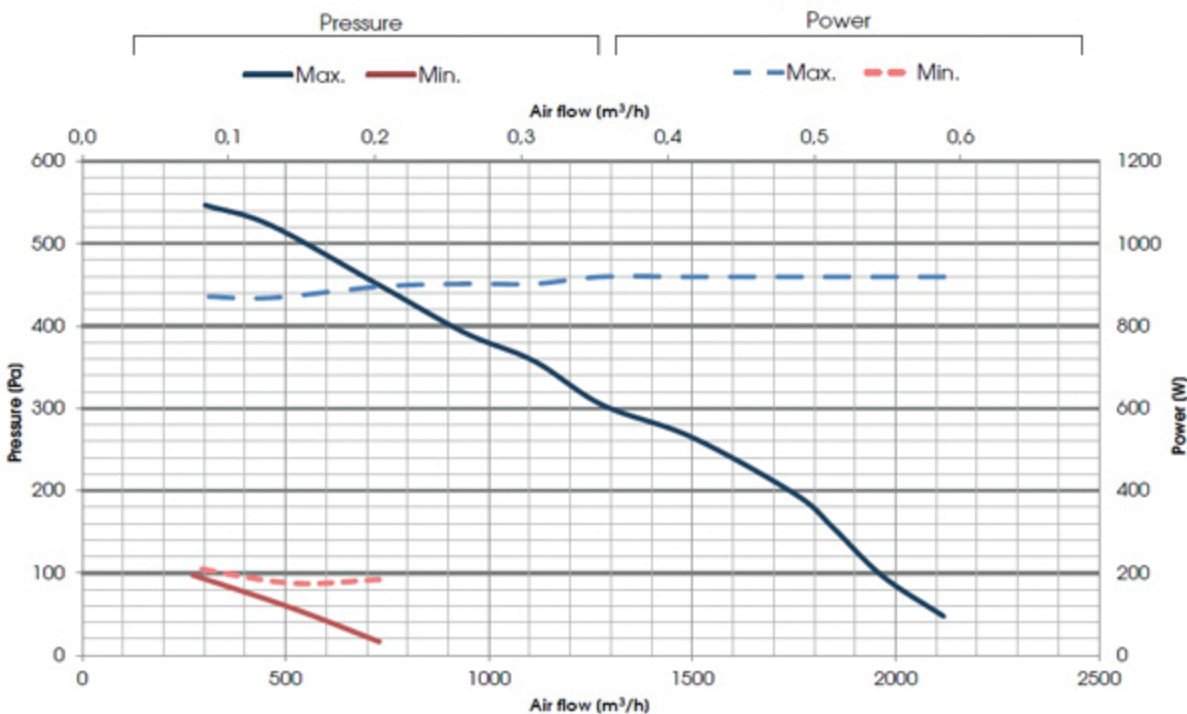
ROTOR H-EC 2 Variable Air Volume (VAV)
