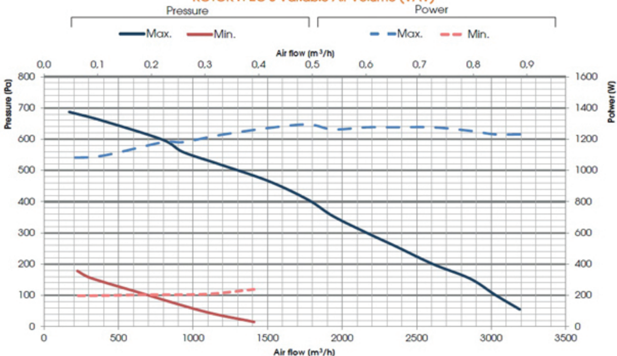
ROTOR H-EC 3 Variable Air Volume (VAV)
