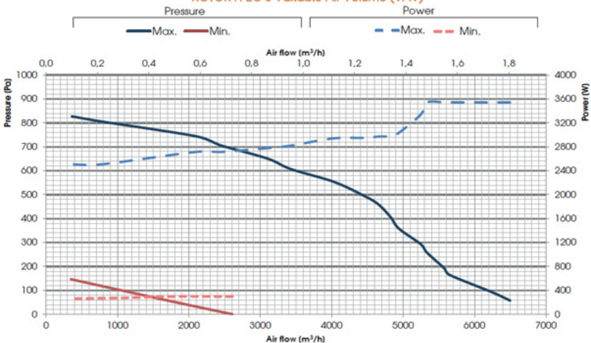
ROTOR H-EC 5 Variable Air Volume (VAV)
